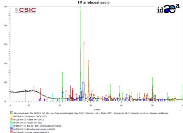
1.- Difractograma d'un arrebossat masnoví.
