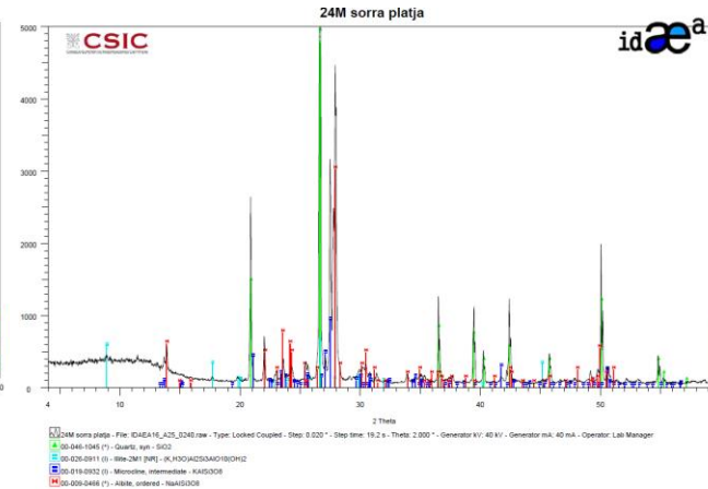
2.-Difractograma de la sorra de platja.
